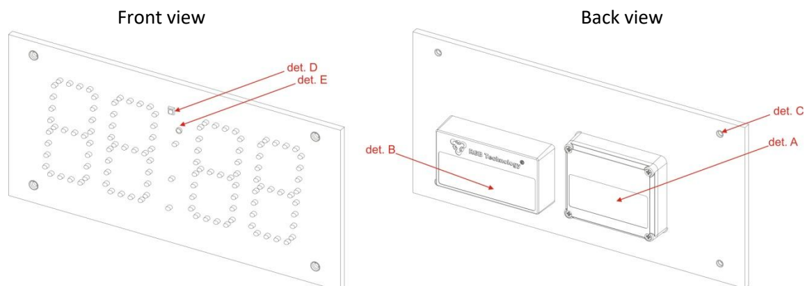
det. A - extender box; det. B - power supply unit; det. C - mounting hole; det. D - IR sensor; det. E - lighting sensor; fig. 1
